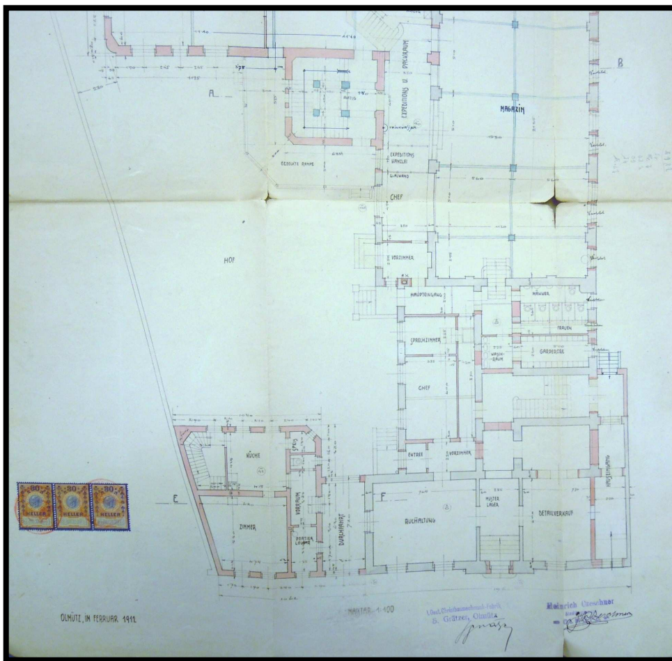
Příloha č. 6: Návrh rozsáhlé přestavby z roku 1912, která nakonec nebyla realizována. Přední část domu od dnešní Palackého ulice – přízemí.
