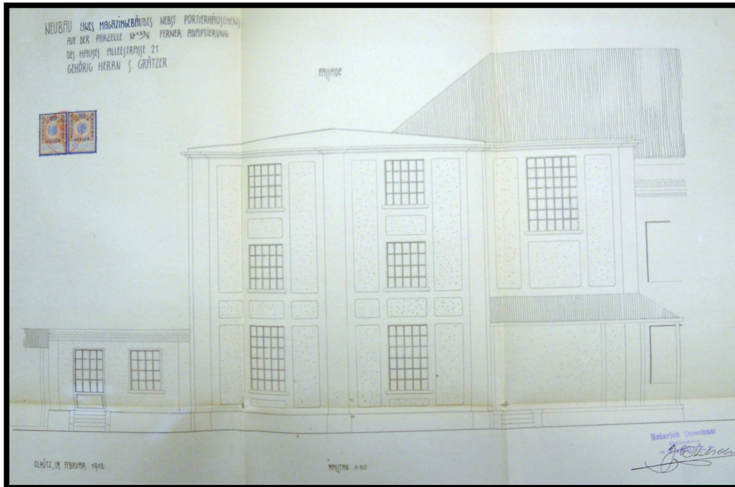
Příloha č. 8: Tentýž projekt – pohled výrobní a skladovací halu od parku, která měla vzniknout ve dvoře.
