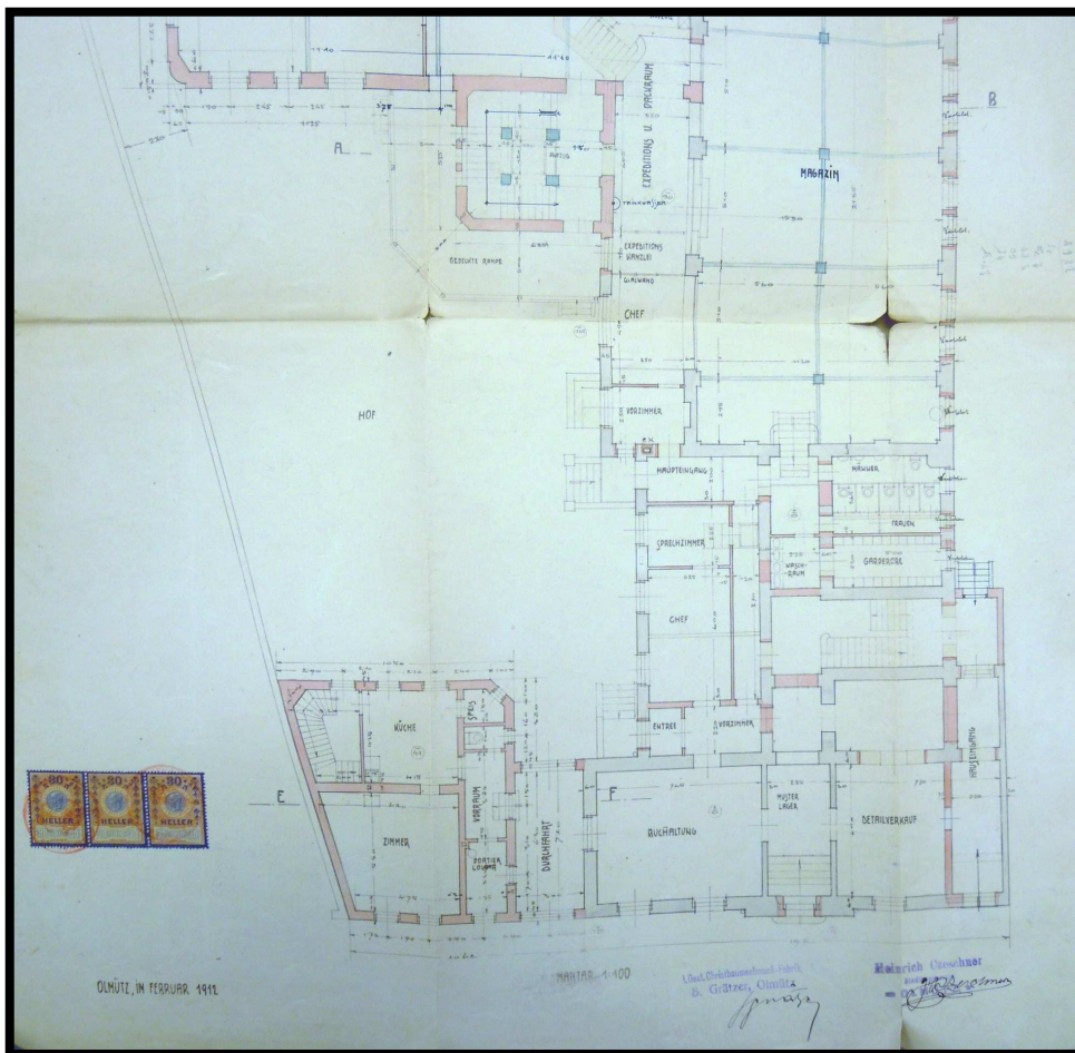
Příloha č. 6: Návrh rozsáhle přestavby z roku 1912, která nakonec nebyla realizována. Přední část domu od dnešní Palackého ulice – přízemí.
